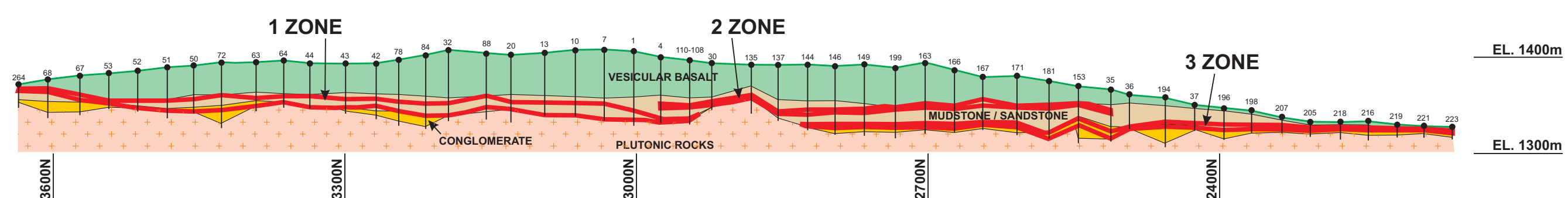
LONGITUDINAL SECTION
